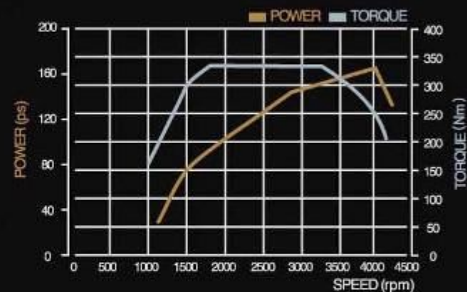
RX270XDi 165ps (121kW) 2,696cc
